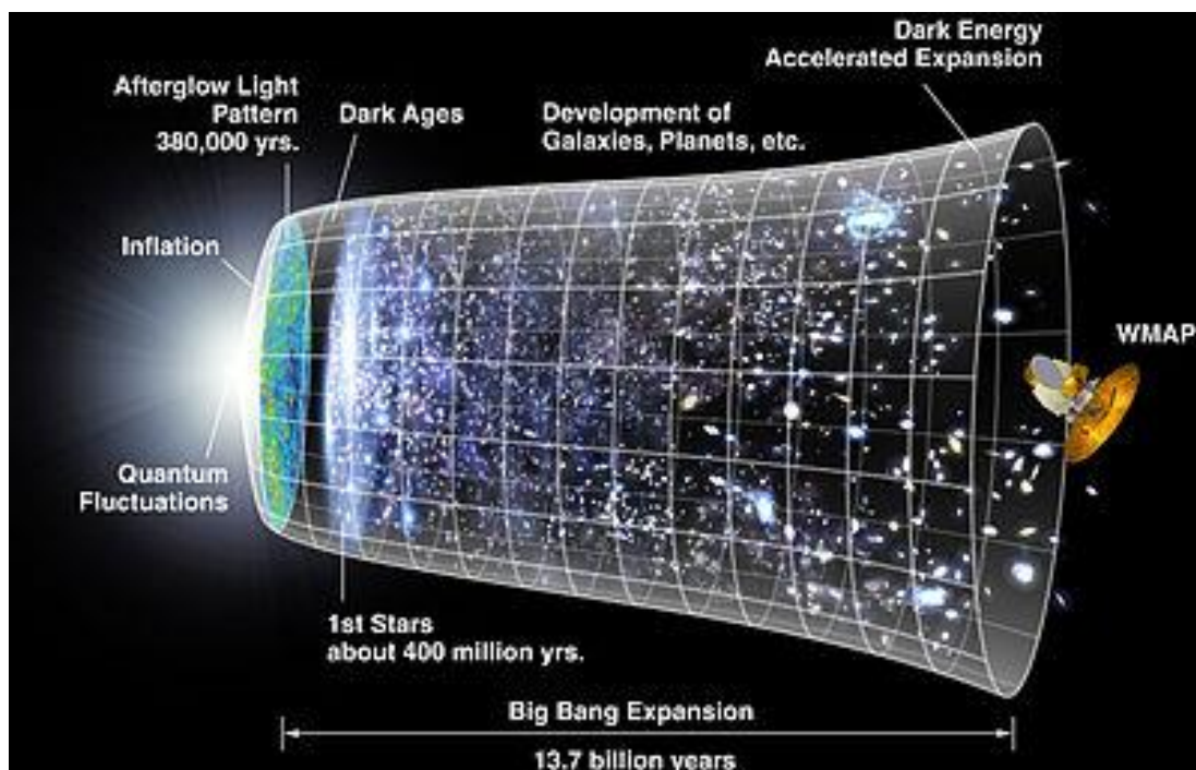
Ontwikkelingsstadia van het universum. Tijd staat op de horizontale as.
